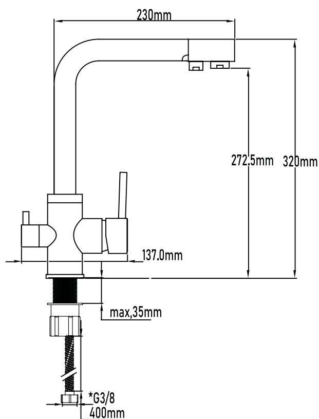
PLANO TÉCNICO
