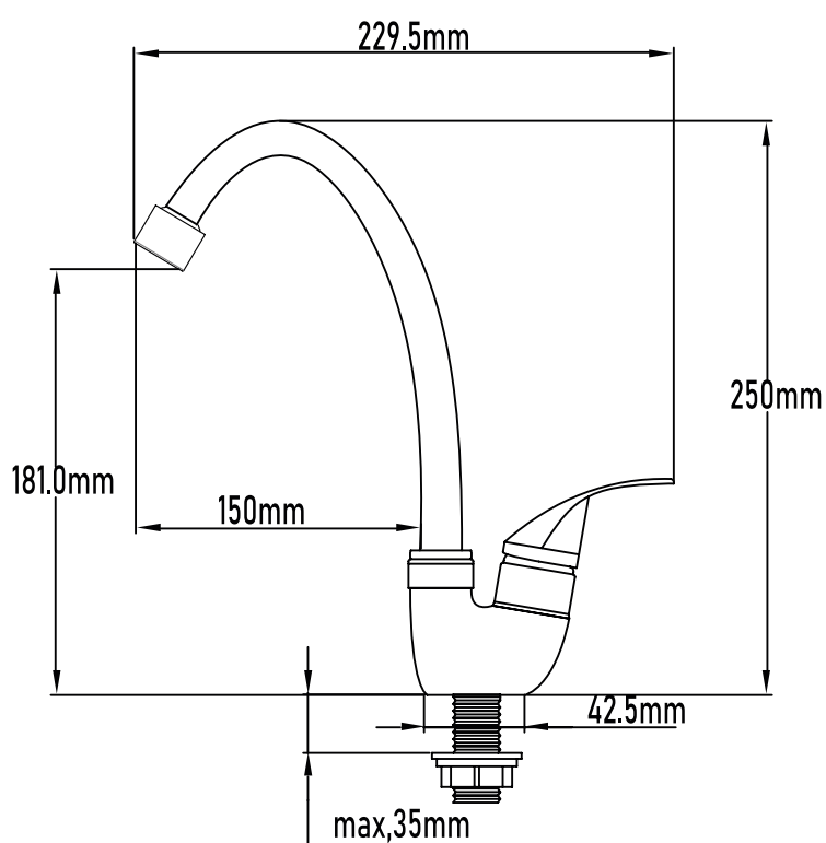
PLANO TÉCNICO
