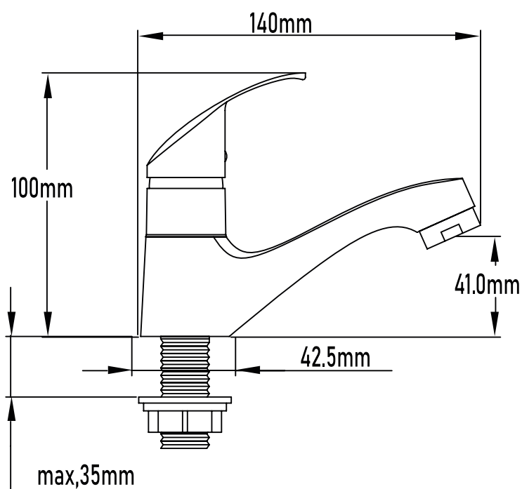
PLANO TÉCNICO
