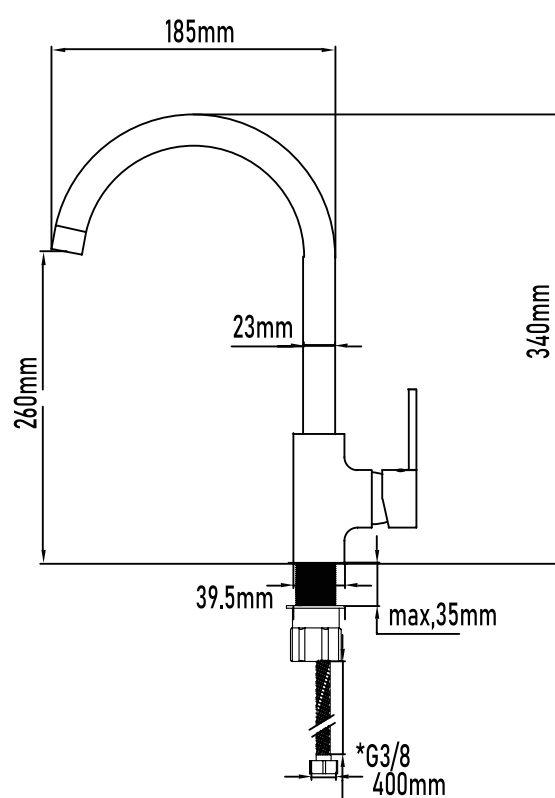
PLANO TÉCNICO
