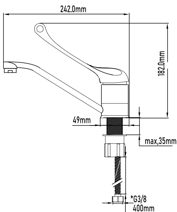
PLANO TÉCNICO
