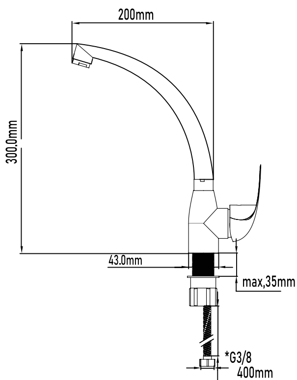
PLANO TÉCNICO
