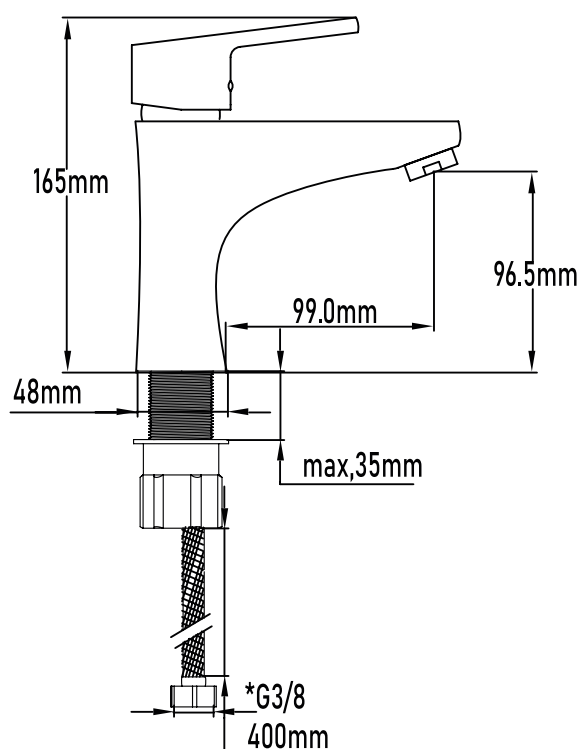
PLANO TÉCNICO
