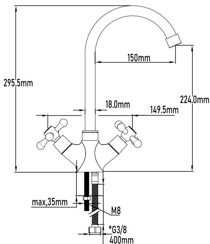
PLANO TÉCNICO
