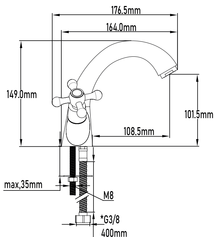
PLANO TÉCNICO
