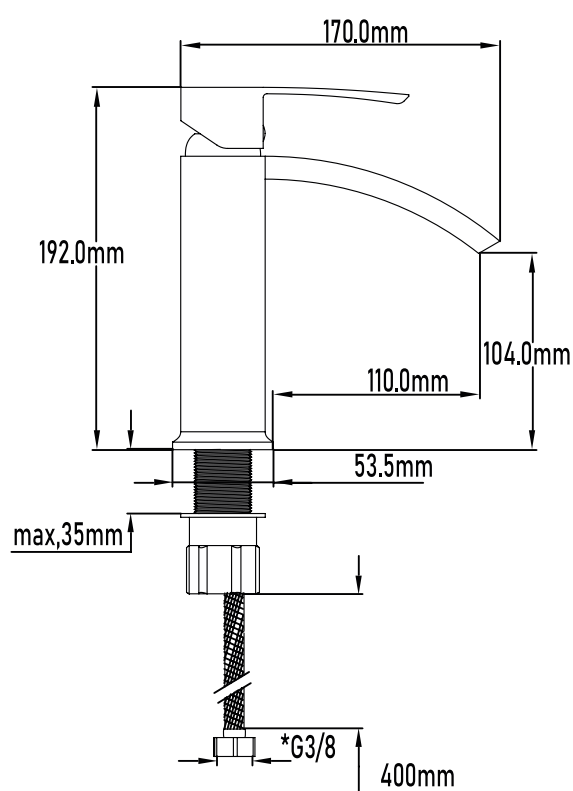
PLANO TÉCNICO
