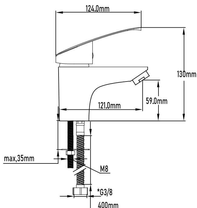
PLANO TÉCNICO
