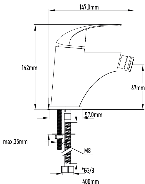
PLANO TÉCNICO
